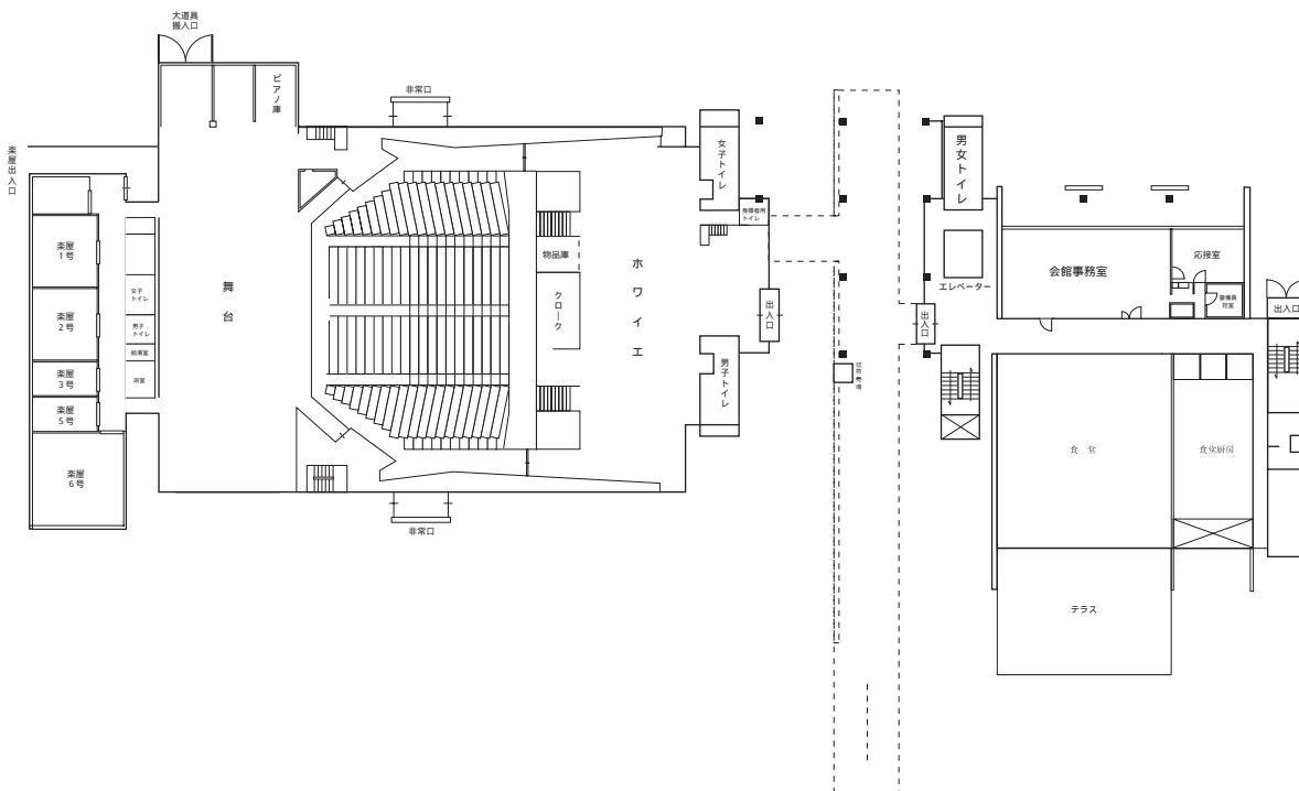
1階平面図
